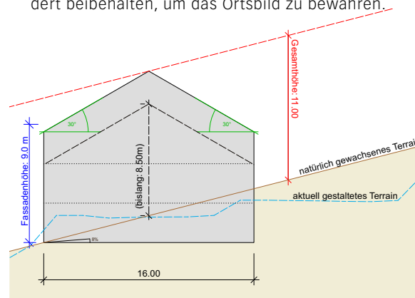
Abb. 8 mögliches Gebäude in der Wohnzone A_1 (Honau)
